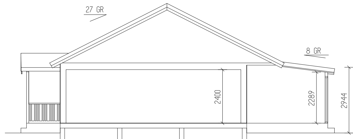
SEKTION A-A
